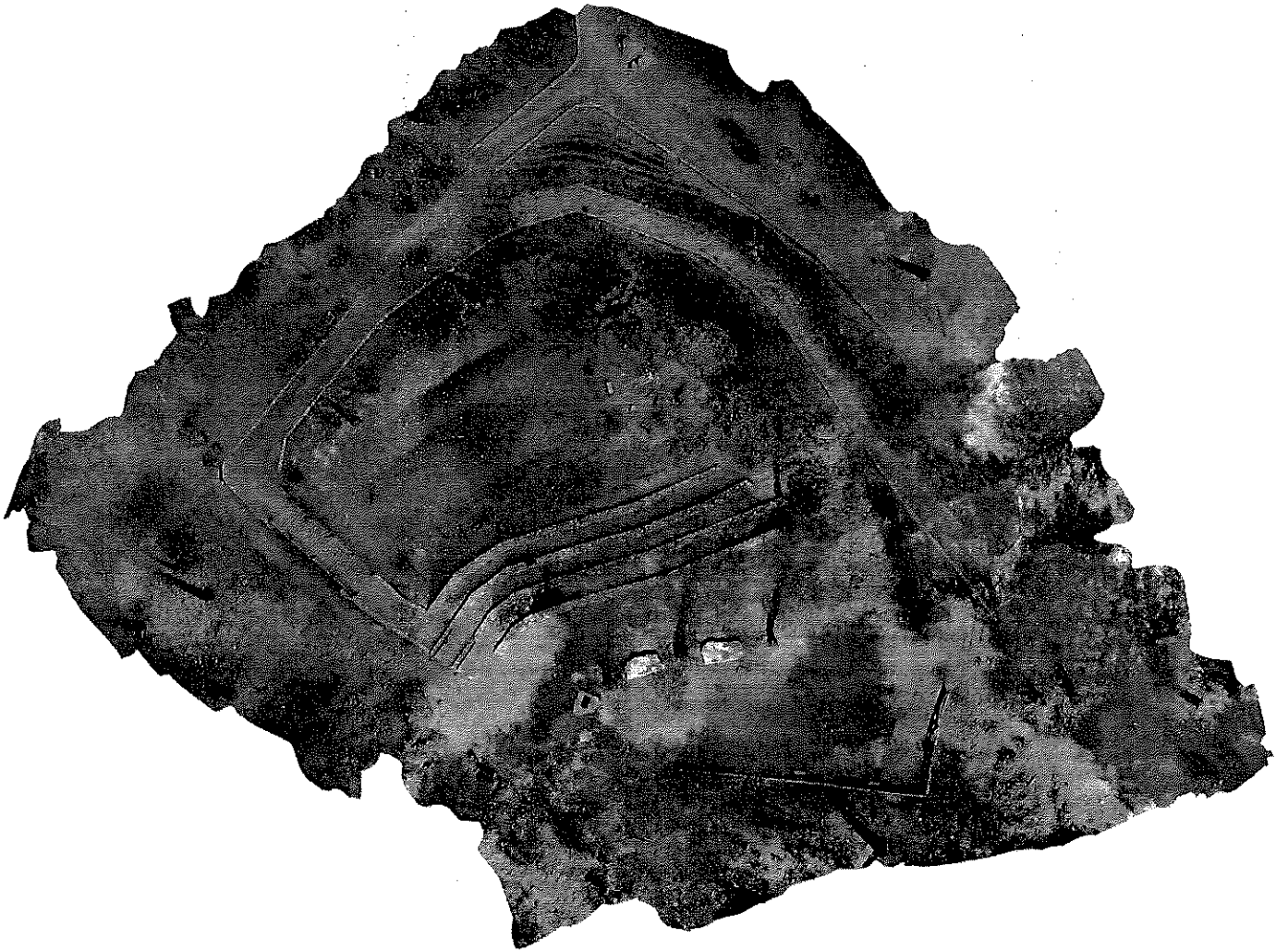
Levantamiento fotogramétrico de detalle del área de intervención con apoyo de puntos de campo colocados mediante estación total
