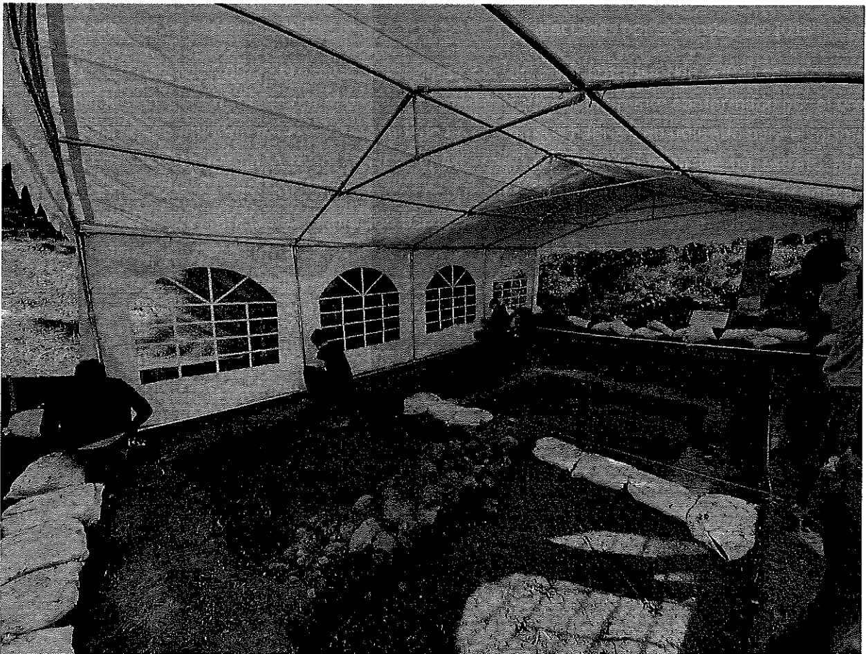
Finalización del montaje del perímetro de control de aguas de escorrentía y de la cubierta.
