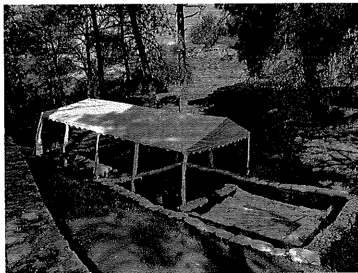
Montaje de perímetro de control de aguas de escorrentía y primeras fases de montaje de la cubierta.
