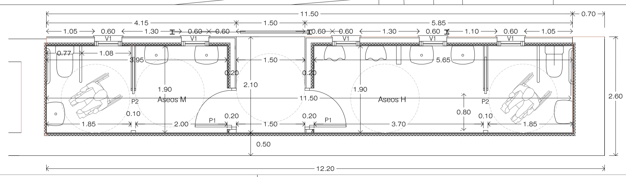
Módulo aseos 1/50
