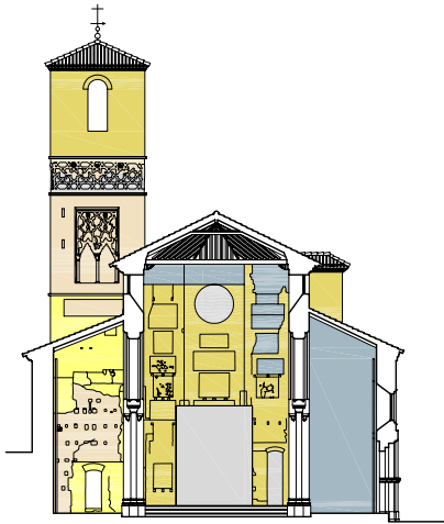
Sección transversal
