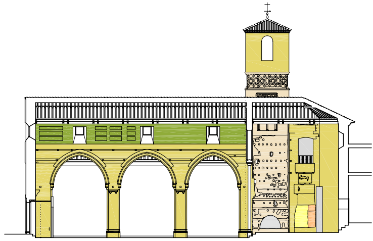
Sección longitudinal
