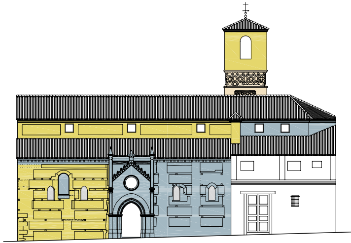
Alzado lateral
